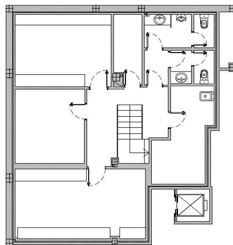
PLANTA SOTANO Superficie: 109,06 m 2 c
